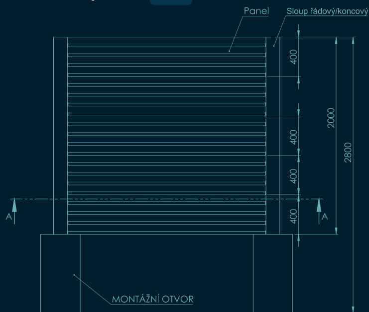
Čelní pohled ALS
