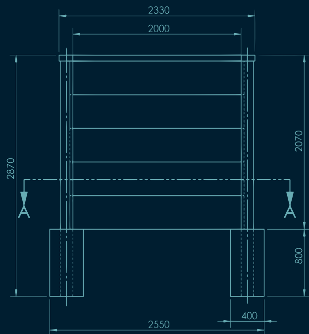
Čelní pohled TVD GR OBR
